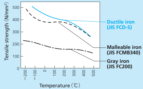
Tensile strength
